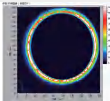
齿轮钎焊C扫描图
