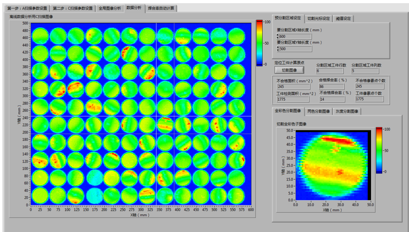
检测报告形式二：一次性检测较大数量工件的 C 扫成像结果
