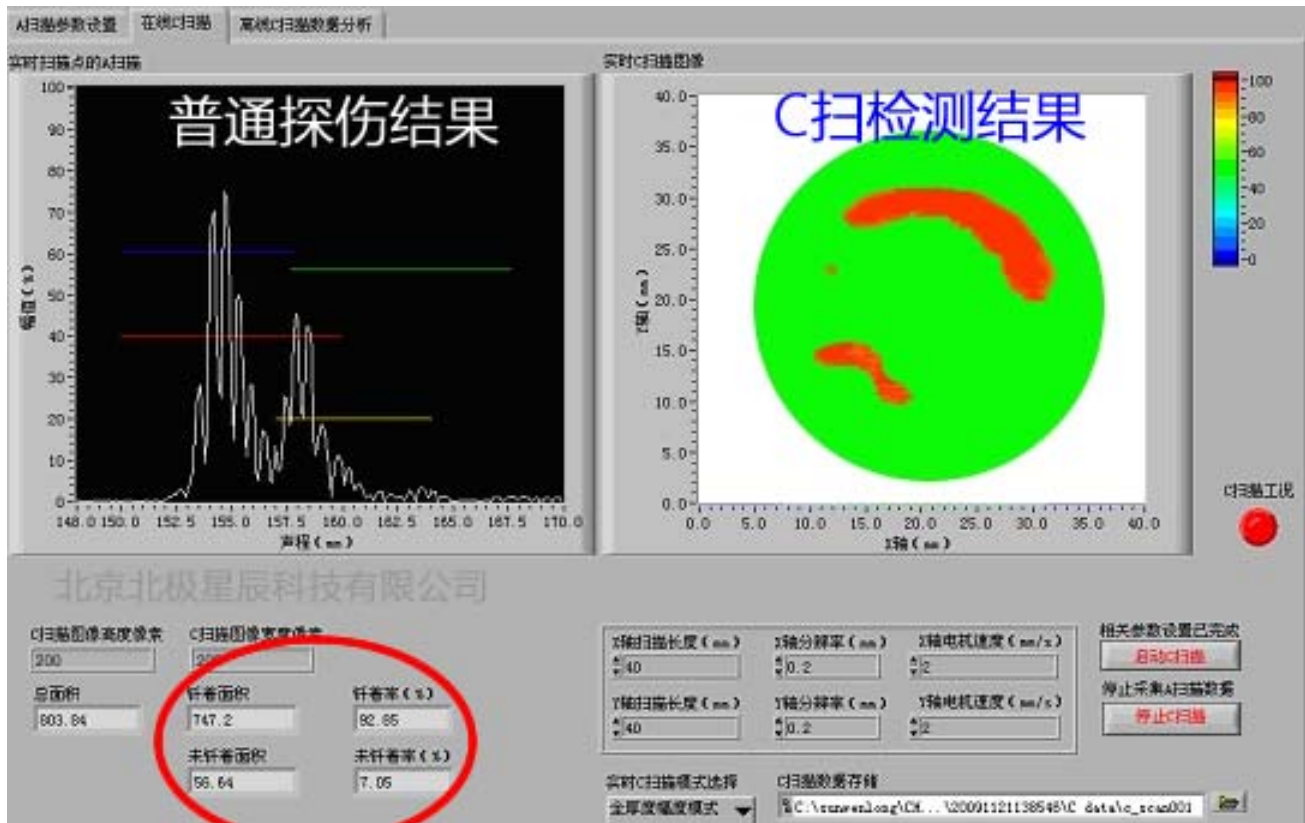
检测报告形式一：单个工件的 C 扫成像结果
